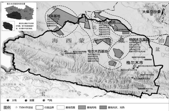
图4-1 “沙戈荒”基地和重点能源项目布局图
